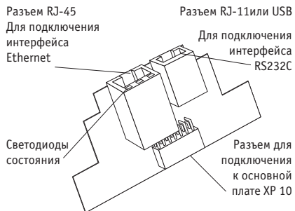
Рис.5 – Общий вид платы интерфейсного submodule WebLinker EM или WebLinker USB
