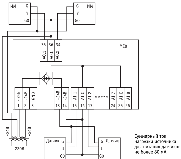
Рис. 9 – Пример подключения цепей питания датчиков 0 -10 В постоянного тока к контроллеру МС8.2х2xxxx
