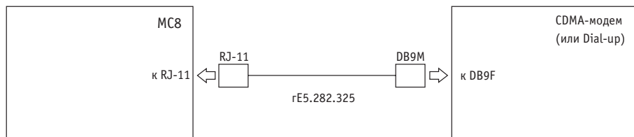
Рис. 16 – Пример подключения контроллера МС8 к CDMA и Dial-up модемам.
