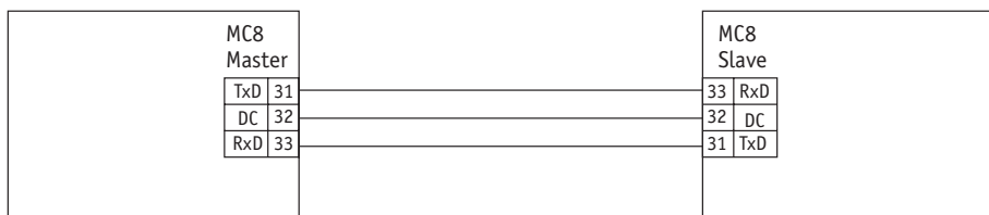
Рис. 12а – Пример подключения 2-х контроллеров МС8.
