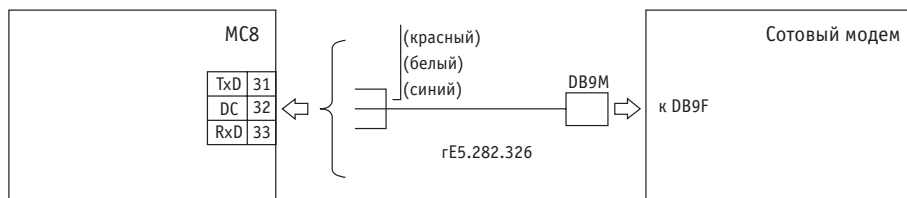
Рис. 12 – Пример подключения сотового модема.
