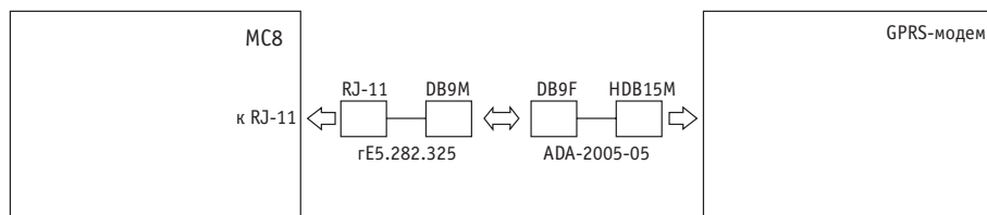
Рис. 15 – Пример подключения контроллера МС8 к GPRS модему.
