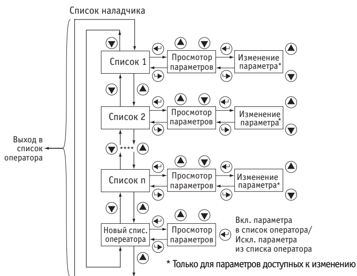
Рис. 19 – Структура меню пульта для списков наладчика
