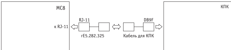
Рис. 14 – Пример подключения контроллера МС8 к КПК по интерфейсу RS232C.
