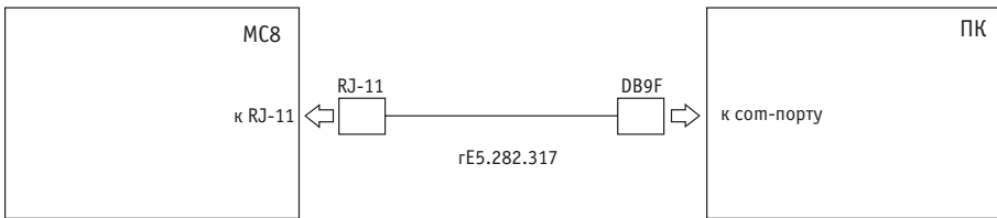
Рис. 13 – Пример подключения контроллера МС8 к ПК по интерфейсу RS232C
